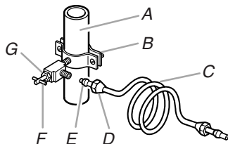
A. Canalisation d'eau froide B. Brique de tuyau C. Tube en cuivre D. Écrou de compression E. Bague de compression F. Robinet d'arrêt G. Écrou de serrage
